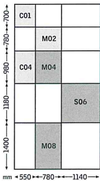
天窓交換用防水シート
